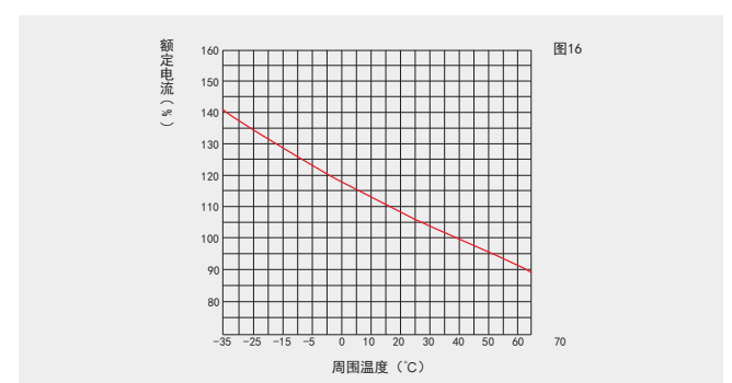
HYM3-800温度补偿曲线
