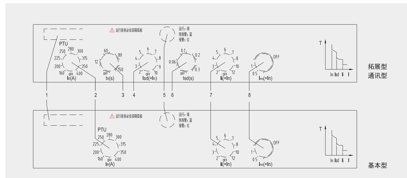
①手持测试单元接口；②过载长延时电流整定；③过载长延时时间整定；④短路短延时电流整定；⑤运行预报警及过电流指示灯 ⑥短路短延时时间整定；⑦短路瞬时电流整定；⑧中性极(N)保护整定(3P无此旋钮)
