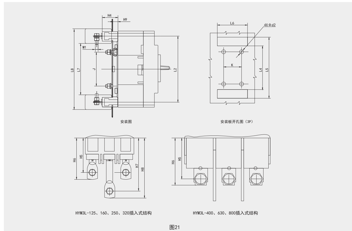
HYM3L系列插入式外形及安装尺寸
