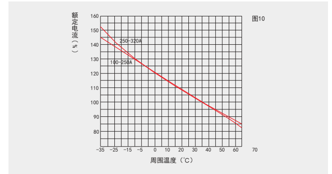
HYM3-400温度补偿曲线
