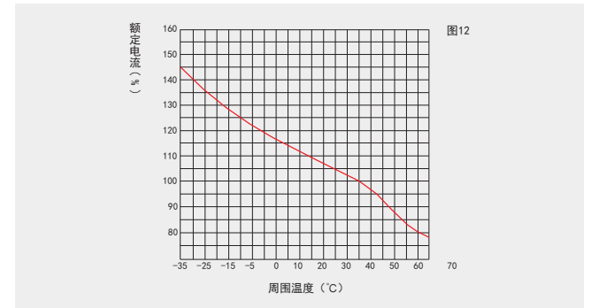
HYM3-630温度补偿曲线
