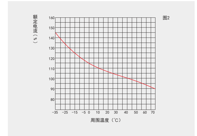
HYM3L-125温度补偿曲线
