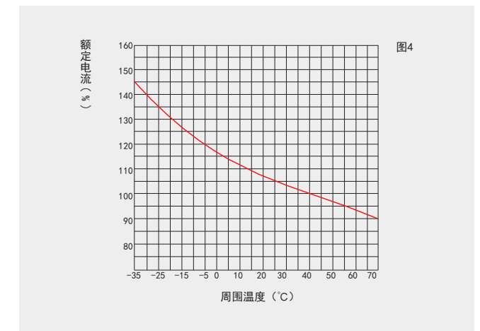
HYM3L-160温度补偿曲线
