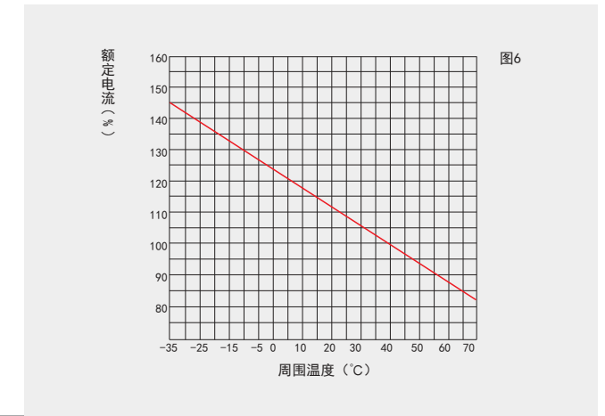
HYM3L-250温度补偿曲线
