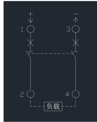
接线图 1
