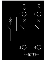
接线图 2
