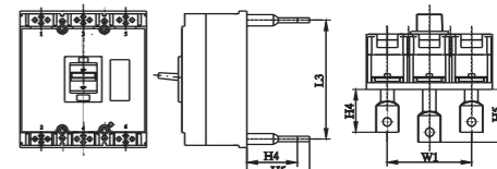
图2 板后接线
