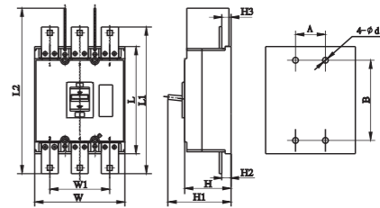
图1 板前接线
